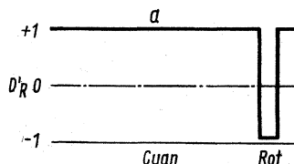
Bild 14a. Möglicher Verlauf der Farbsignalspannung bei richtiger Übertragung der zugehörigen Gleichspannungskomponente. Trennt man die Gleichspannung über einen Kondensator ab, so ergibt sich ein Signalverlauf nach Bild 14b. Man erkennt den wesentlich vergrößerten notwendigen Aussteuerbereich
