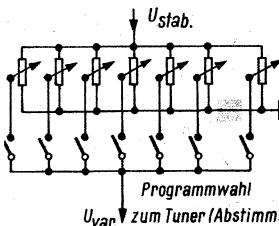
Bild 2. Mechanische und elektrische Ausführung der elektronischen Abstimmung
