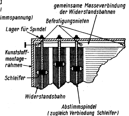
Bild 2. Mechanische und elektrische Ausführung der elektronischen Abstimmung
