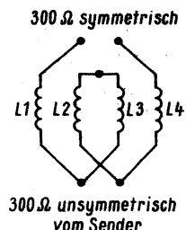
Bild 11. Schaltung eines Hf-Transformators (Balun) für 300-Ω-Eingang (unsymmetrisch) und 300-Ω-Ausgang (symmetrisch)
