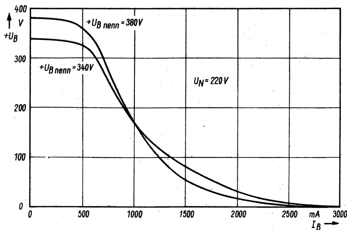
Bild 21. Ausgangsspannung als Funktion des Laststromes (bis zum Kurzschluß)
