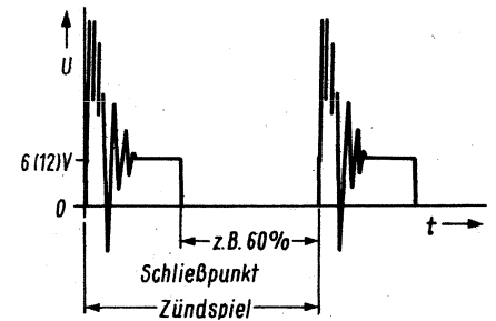
Bild 1. Oszillogramm der Spannung am Unterbrecherkontakt (bzw. Punkt 1 der Zündspule)
