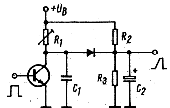
Bild 4. ▶ Schaltung zur Erzeugung von Kennimpulsen
