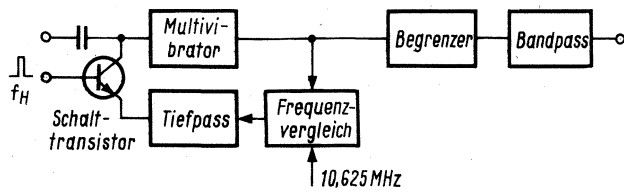
Bild 7. Blockschaltbild eines Frequenzmodulators
