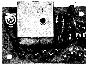
Görler-Rauschperre (14) »Typ 326-0010«
