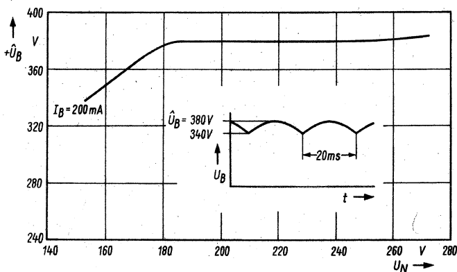
Bild 23. Ausgangsspannung des Netz teiles mit Modulator als Funktion der Netzspannung
