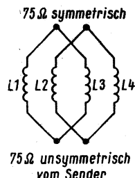
Bild 10. Schaltung eines Hf-Transformators (Balun) für 75-Ω-Eingang (unsymmetrisch) und 75-Ω-Ausgang (symmetrisch)
