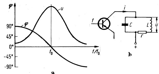
Bild 2. a = Amplituden- und Phasenverlauf eines Schwingkreises; b = Meßanordnung (Ausgangswiderstand des Transistors vernachlässigt)
