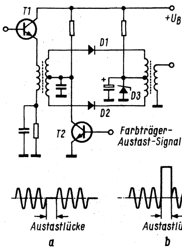
Bild 12. Austastung des Farbsignals. a = Austastung nur der Wechselspannung, b = Austasten der Wechselspannung bei gleichzeitiger Änderung des Arbeitspunktes
