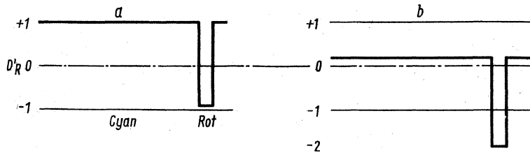
Bild 14a. Möglicher Verlauf der Farbsignalspannung bei richtiger Übertragung der zugehörigen Gleichspannungskomponente. Trennt man die Gleichspannung über einen Kondensator ab, so ergibt sich ein Signalverlauf nach Bild 14b. Man erkennt den wesentlich vergrößerten notwendigen Aussteuerbereich
