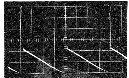
Bild 18. Vertikalfrequente Eingangsspannung des Modulators (Punkt A). Maßstab: vertikal 10 V/T, horizontal 5 ms/T
