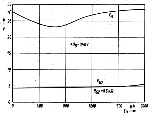
Bild 24. Anoden- und Schirmgitterverlustleistung einer Röhre PL 509 in einer mit diesem Netzteil betriebenen Horizontal-Endstufe für 110°-Farbbildröhre in Abhängigkeit vom Strahlstrom
