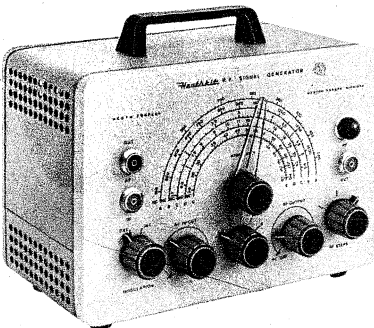
Universal-Prüfender SG-9*
