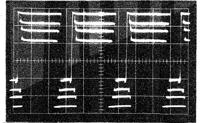
Bild 13. Spannung an der Anode des Thyristors GTO bei 0, 100, 200, 300 mA Laststrom. Maßstab: vertikal 100 V/T, horizontal 20 \mu s/T
