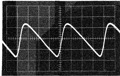
Bild 15. Restbrümm am Kondensator C 5 bei Belastung mit etwa 80 W. Maßstab: vertikal 5 V/T, horizontal 5 ms/T
