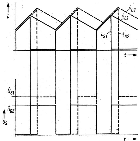
Bild 2. Strom, der über den Schalter S fließt
