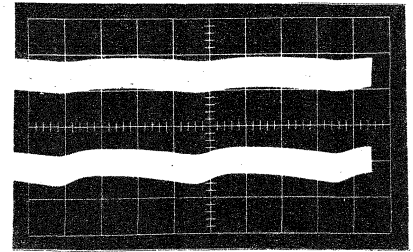
Bild 16. Netzfrequenter Restbrümm am Ausgang des Netzteiles bei 80 W Belastung. Maßstab: vertikal 1 V/T, horizontal 5 ms/T
