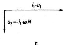
Bild 4. a = Bandfilter mit induktiver Kopplung M ; b = Ersatzschaltung für den zweiten Kreis; c = Zeigerdiagramm
