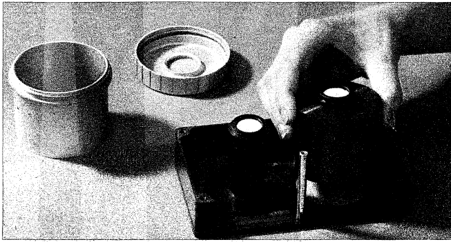
▲ Bild 1. Diese kleine Ampex-Kassette nimmt ein 2-Zoll-Magnetband für eine Spielzeit von 10 s auf, ausreichend für Werbespots oder sonstige kurze Einblendungen in das Fernsehprogramm. Bei Nichtgebrauch oder für den Postversand wird der Bandwinkel in dem leichten Behälter links untergebracht
