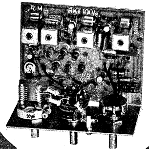
RIM-KW-Super (12) »RKT 100 S«
