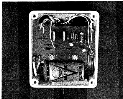
Bild 4. Innenaufbau des Schließwinkelmeßgerätes
