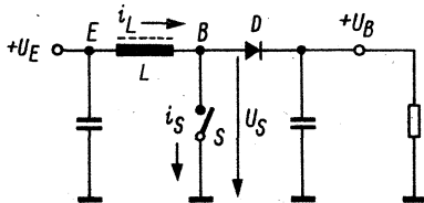
Bild 1. Prinzipschaltung des Netztesles
