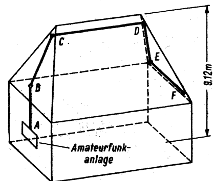
Bild 2. Langdrahtantenne für Dachbodenmontage mit Ableitung an der Gebäude-Stirnseite
