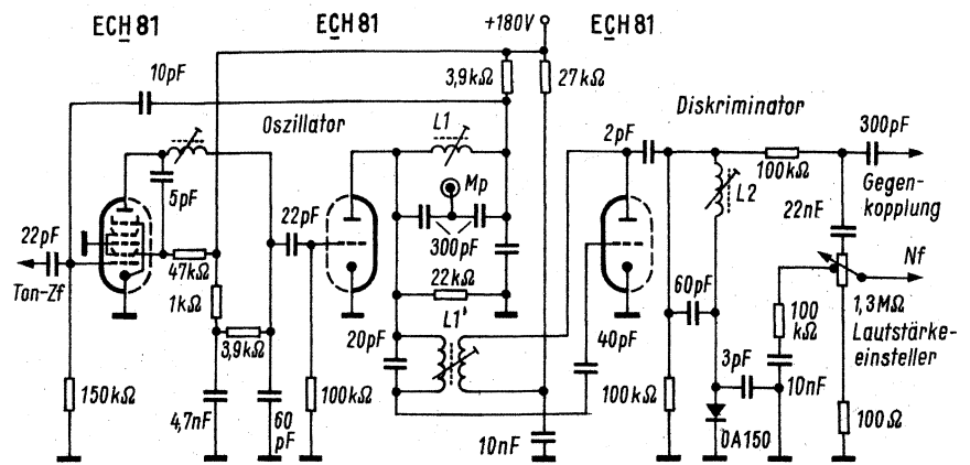
Durch einen Fehler im Synchro-Oszillator – der Kern der Oszillatorspule L1 bestand nur noch aus kleinen Bröckchen – fehlten Bild und Ton
